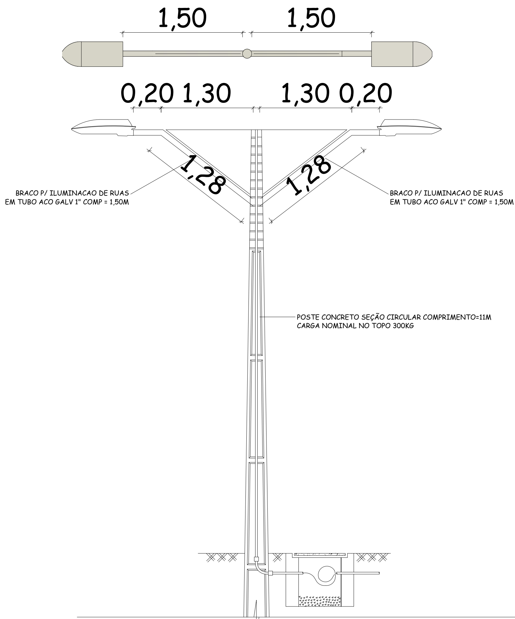
Detalhamento dos postes Escala SN
