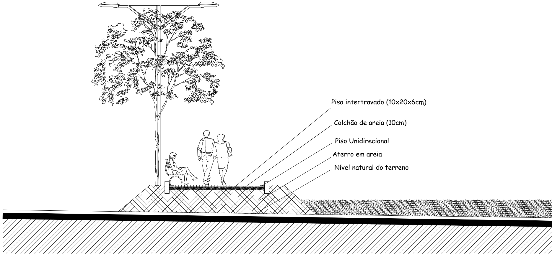
Corte X X' Escala 1:75
