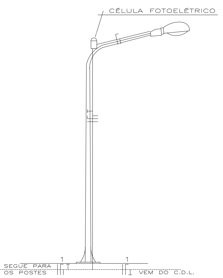
DETALHE RELÉ FOTOELÉTRICO Sem escala
