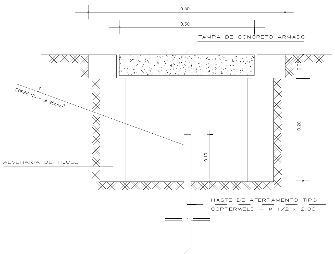
DET. DA CX. DE ELETRODO DE ATERRAMENTO SEM ESCALA
